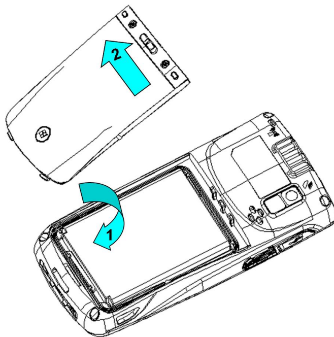
图 1-5 安装电池
